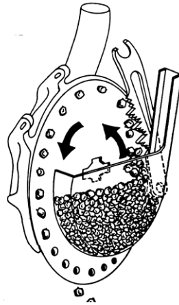
جهاز التلقيح بقوة سحب الهواء.
