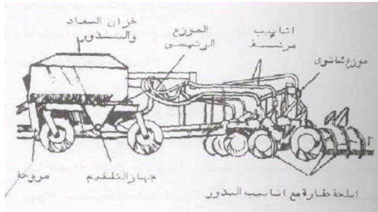
أجزاء آلة تسطير البذور الهوائية.
