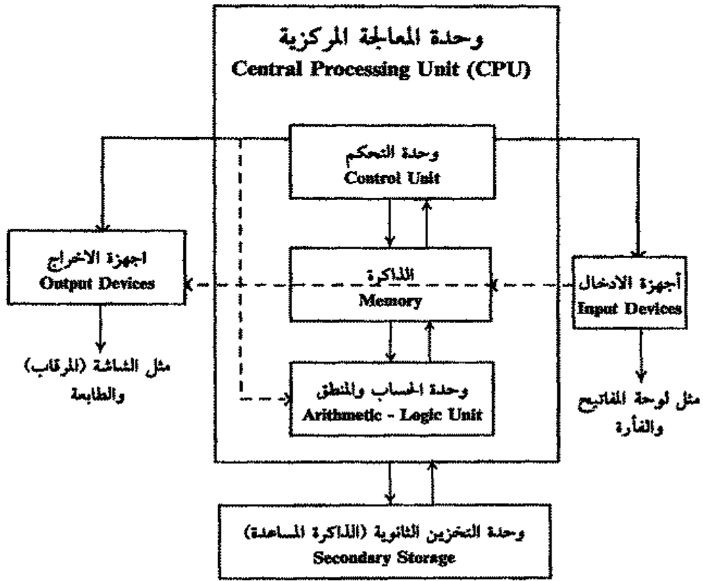
المكونات المادية للحاسبات الآلية (شكل مكونات مادية - ٤)
