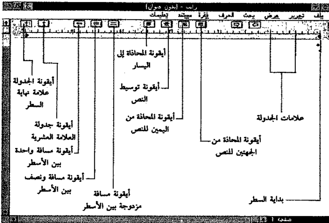
الشاشة الأولى لبرنامج الكتابة العربية Arabic Write شكل (ويندوز - ٦).
