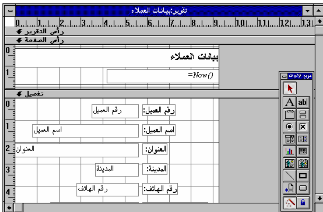
شكل (77) نافذة تصميم التقرير
