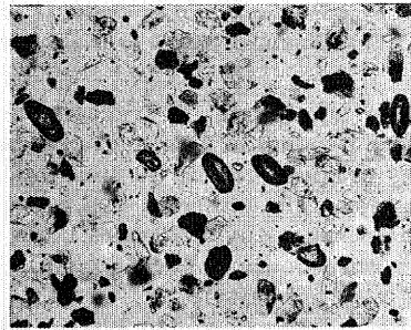
f) Fracción -270.-m Aparición de cristales partidos
