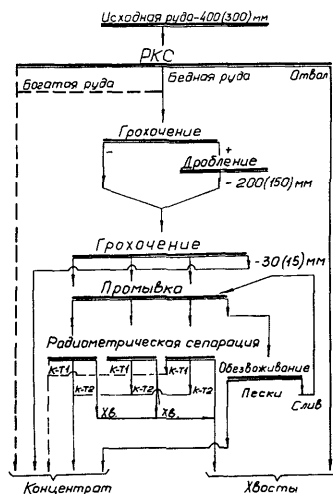
Рис. 1. Типовая схема радиометрической обогатительной фабрики.
