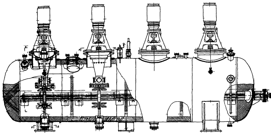
Рис. 2. Автоклав для выщелачивания бедных урановых руд.
