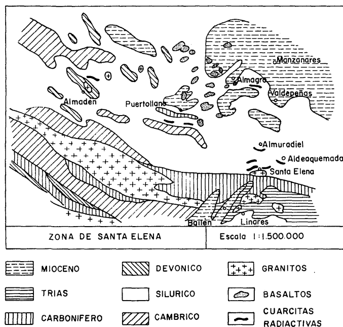
FIG. 1.- Mineralizaciones de circón más importantes en España y detalle de los afloramientos de las cuarcitas de la zona de Santa Elena.
