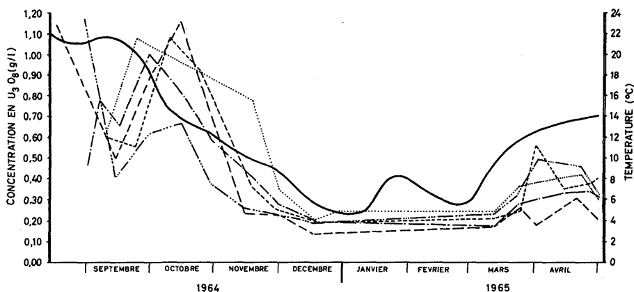
FIG. 4. Concentration des liqueurs et température moyenne de l'air.
