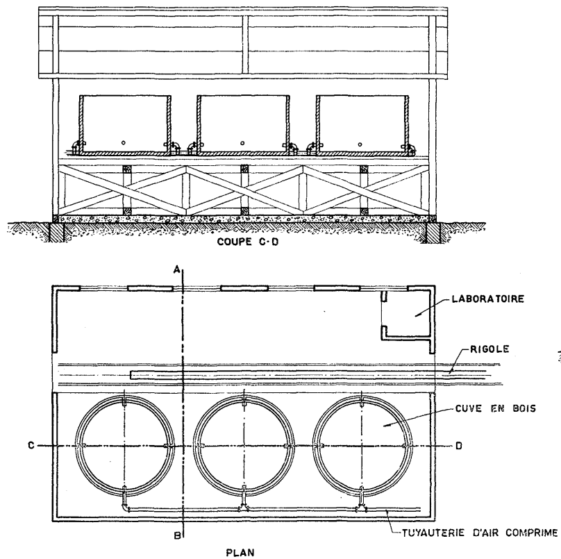
FIG. 7. Atelier de précipitation.
