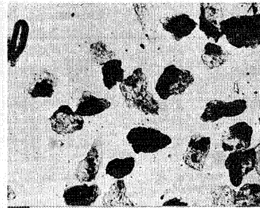
d) Fracción -150+200.-m. Abundancia de circón liberado junto a mixtos
