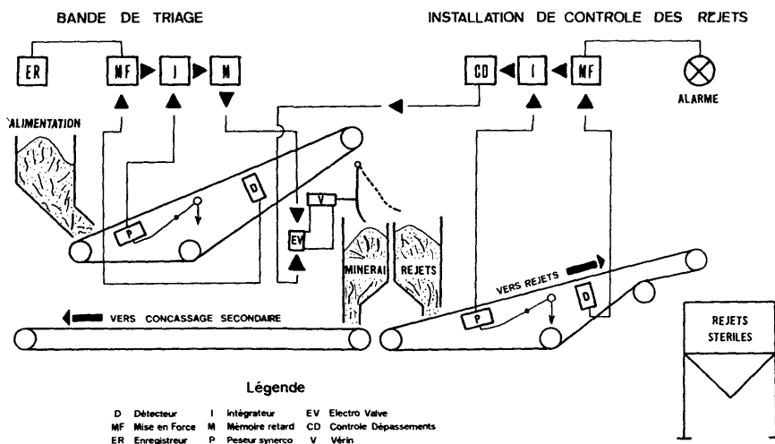
FIG. 2. Atelier de préparation des minerais de Bessines.
