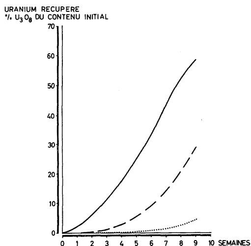
FIG. 3. Minerais à faible teneur en uranium: rendement d'extraction (essais à petite échelle).
